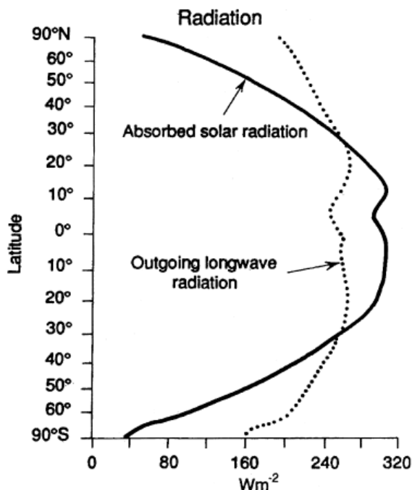
Figuur 2. Weergave van het energiebudget van de aarde op verschillende geografische breedtes
