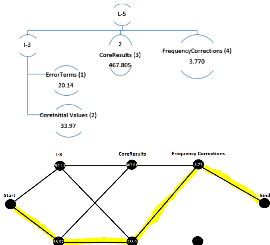
Figuur 17. Lineair CLAN en de beslissingsgraaf
