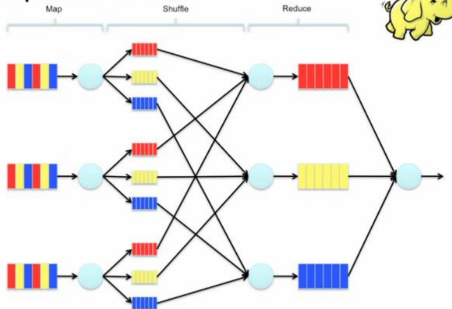
Figuur 4. MapReduce schema
